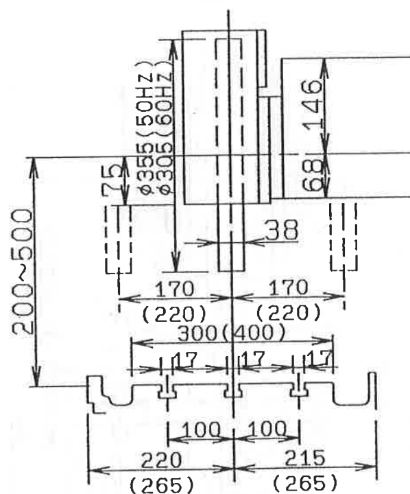
加工範囲図
